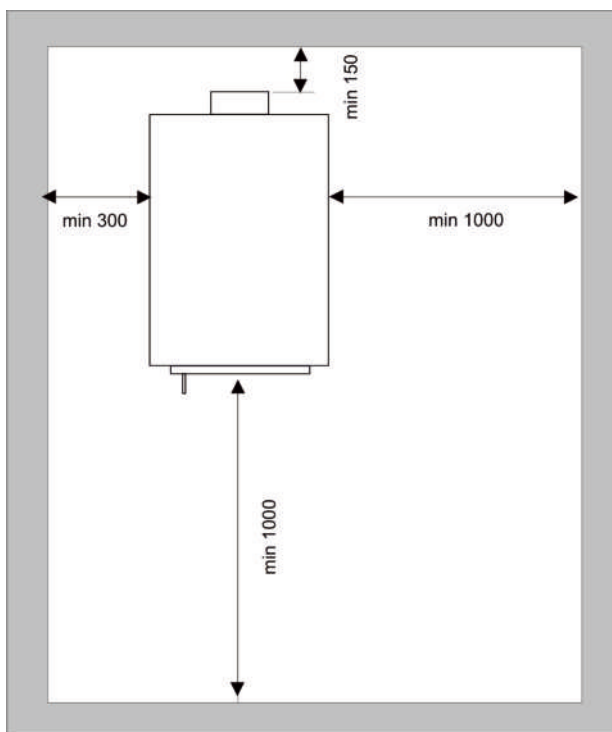
Мал. 3 - Схема правильного розташування котла в приміщенні
