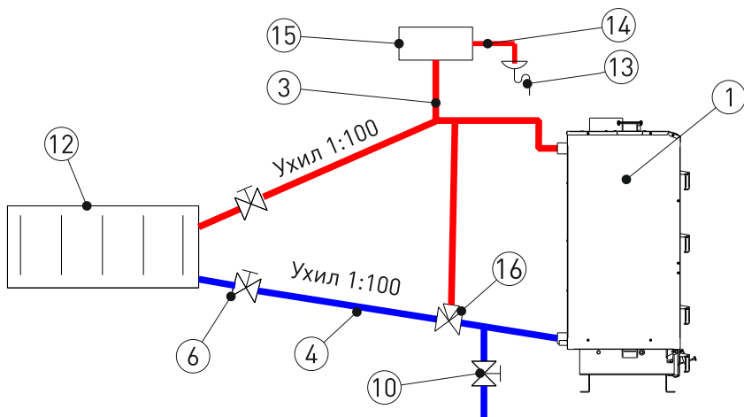
Малюнок 4.2 - Схема відкритої системи опалення
